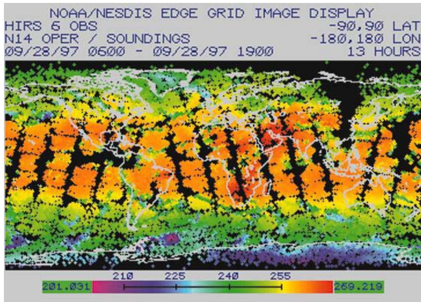
Fig.3 - Temperatura atmosférica global procedente do canal 6 do HIRS do satélite NOAA 14
