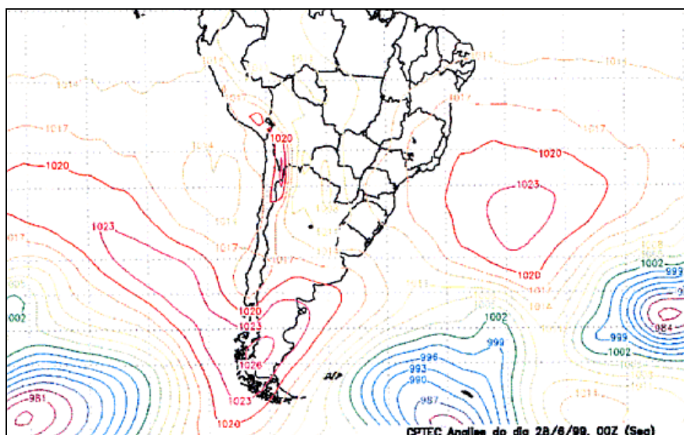
Fig. 5 - Análise do dia 28 / 06 /1999 00 GMT - Modelo Global CPTEC
