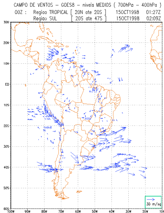
Fig. 4 - Campo de ventos obtidos a partir de imagens do GOES 8
