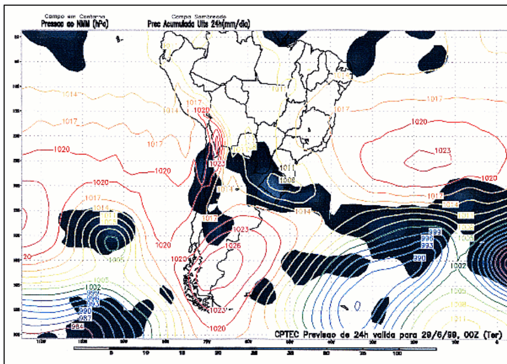
Fig. 6 - Previsão de 24 horas Válida para 29/ 06/ 1999 00 GMT
