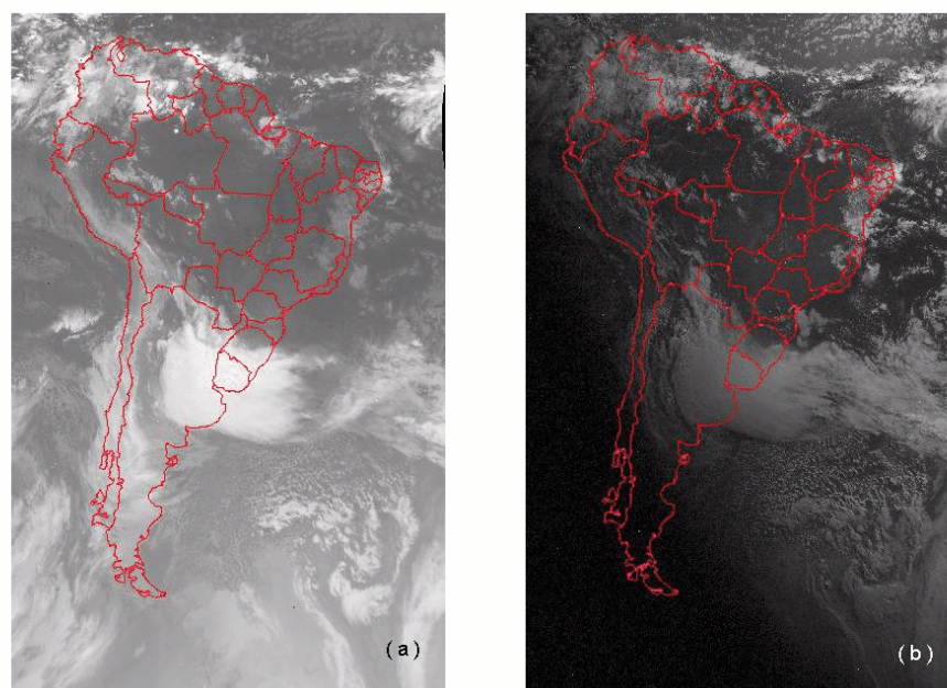
Fig. 2 - Imagem GOES 8 de 28/06/99 12:00 UTC nos canais: (a) Infravermelho ; (b) Visível
