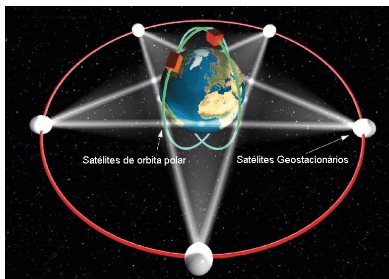
Fig. 1 – Visão esquemática das órbitas dos satélites meteorológicos operacionais.
