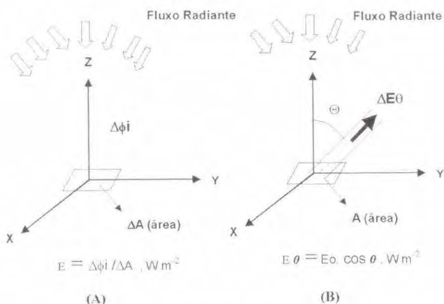
Fig.6.4 – Esquema para ilustrar a irradiância – E (A) e a lei do co-seno da irradiância (B). FONTE: adaptada de Steffen et al. (1996)
