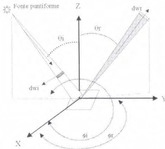
Fig. 7.1 – Geometria do fluxo incidente e do refletido pelo alvo. Onde, i e r são os fluxos incidentes e refletidos, dwi e dwr são os ângulos sólidos, dA é a unidade de área imageada, \theta é o ângulo azimutal e \phi é o ângulo zenital em relação ao eixo Z, perpendicular à área dA . FONTE: adaptada de Nicodemus et al. (1977).
