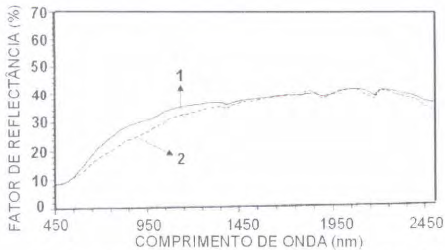
Fig. 3.21 - Curvas espectrais para amostras de Solos Areias Quartzosas descritas na Tabela 3.9.
