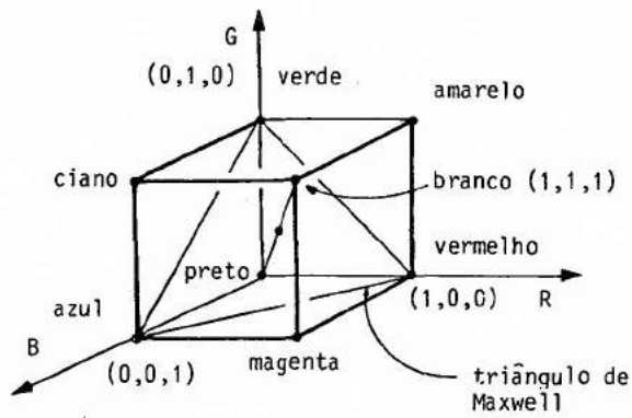
Figura 8.6 Cubo RGB.
