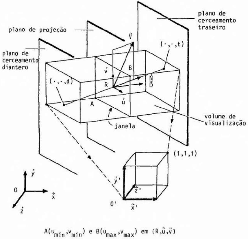
Figura 3.4 Mapeamento do volume de visualização para o cubo unitário.
