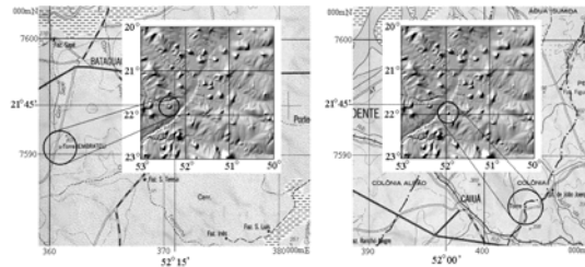
Figura 1. Correspondência entre os artefatos na imagem (detalhe) e a presença de torres: torre Embratel, município de Bataguáçu (esq.); torre no município de Caiuá (dir.). Folha IBGE (1:250000) SF-22-V-D
