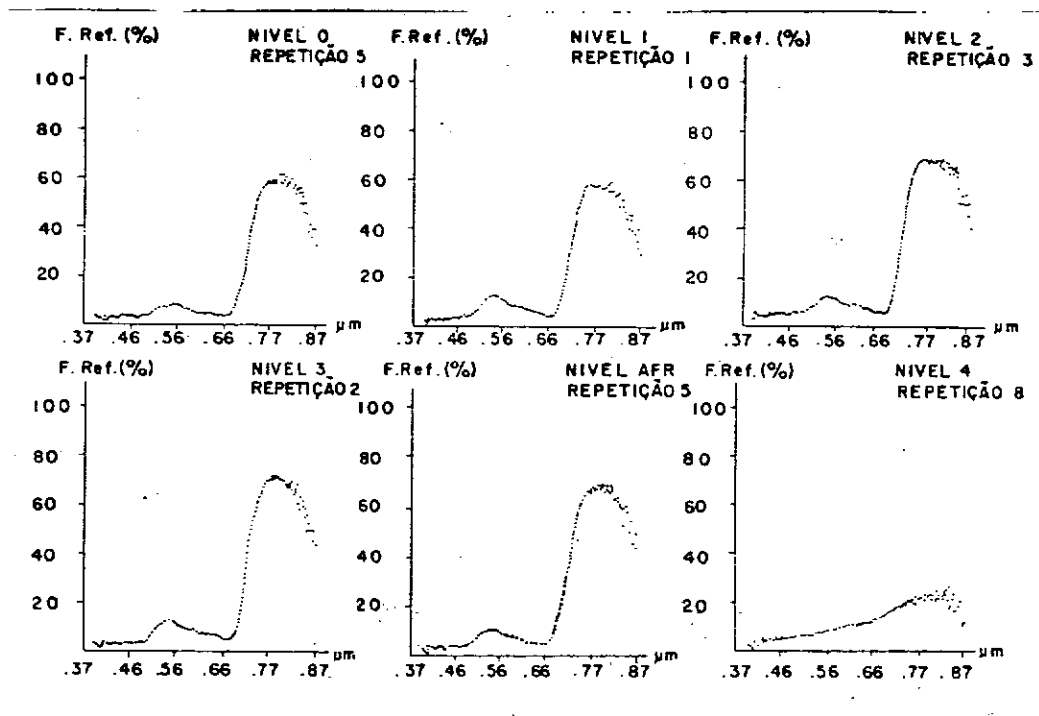
Fig.22 - Reflectância das acículas de Araucaria provenientes de indivíduos que apresentavam diferentes níveis de danos.
