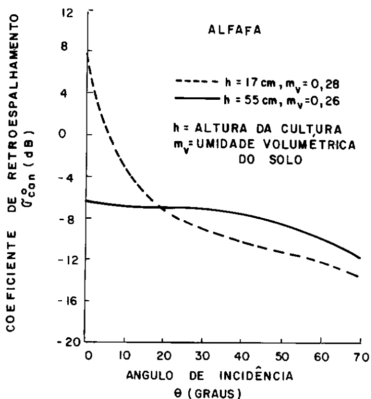
Figura 18 - Coeficiente de retroespalhamento da cultura de alfafa em duas fases de crescimento.
