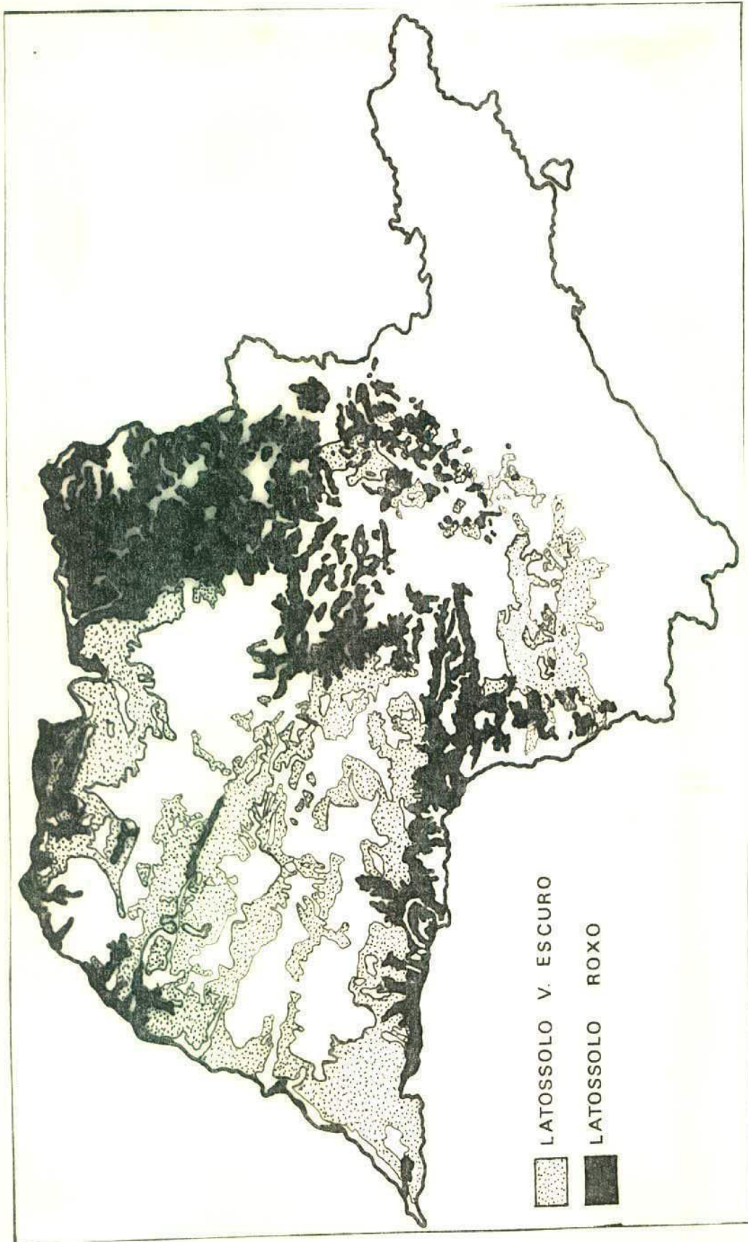
Fig. II.2 - Mapa Esquemático da Localização das Duas Classes de Solos Estudadas. Fonte: Levantamento de Reconhecimento dos Solos no estado de São Paulo, 1960.
