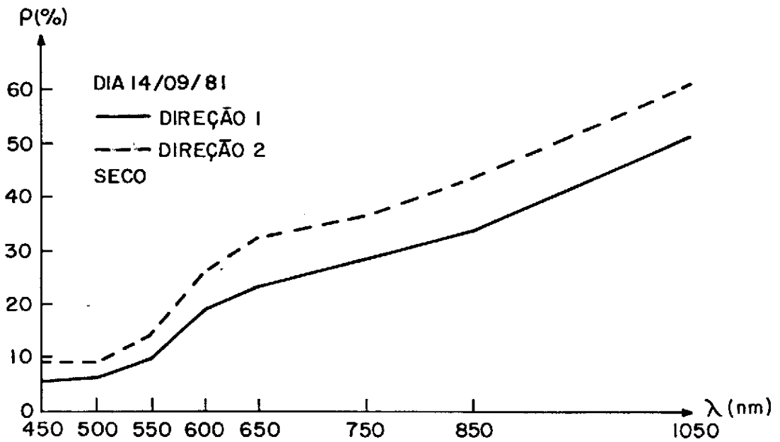
Fig. 3.4 - Comportamento espectral da parcela seca segundo as direções de observação 1 e 2 (14/9/81).
