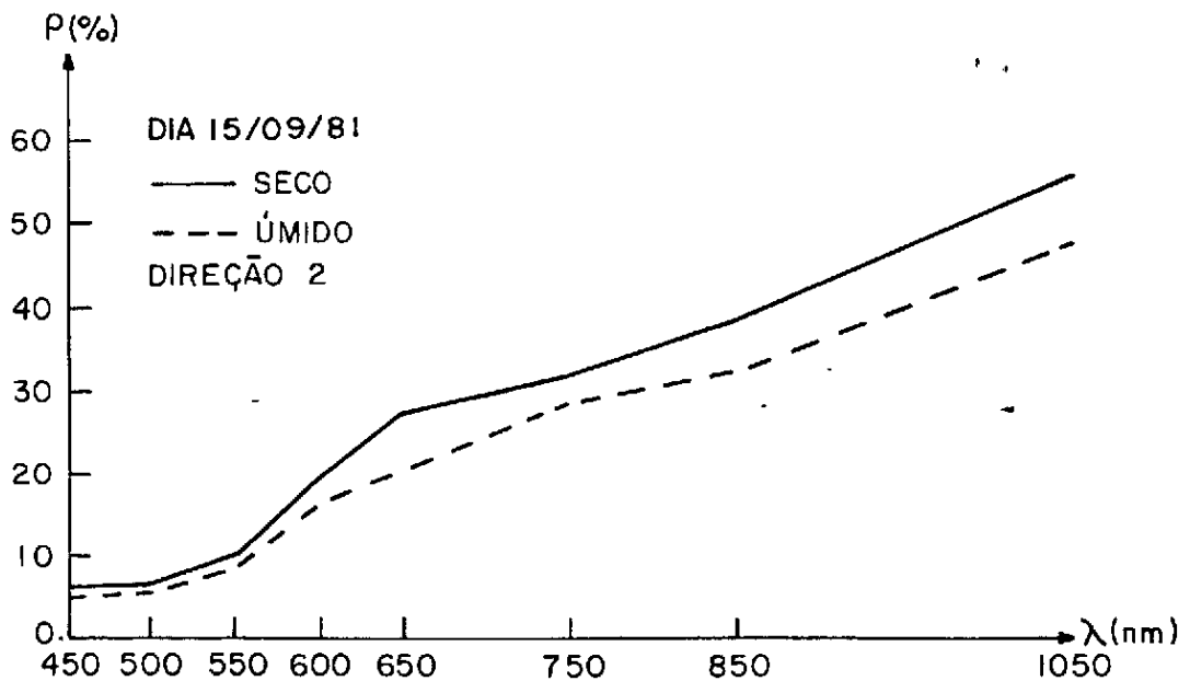
Fig. 3.21 - Comportamento espectral das parcelas seca e úmida segundo a direção de observação 2 (15/9/81).
