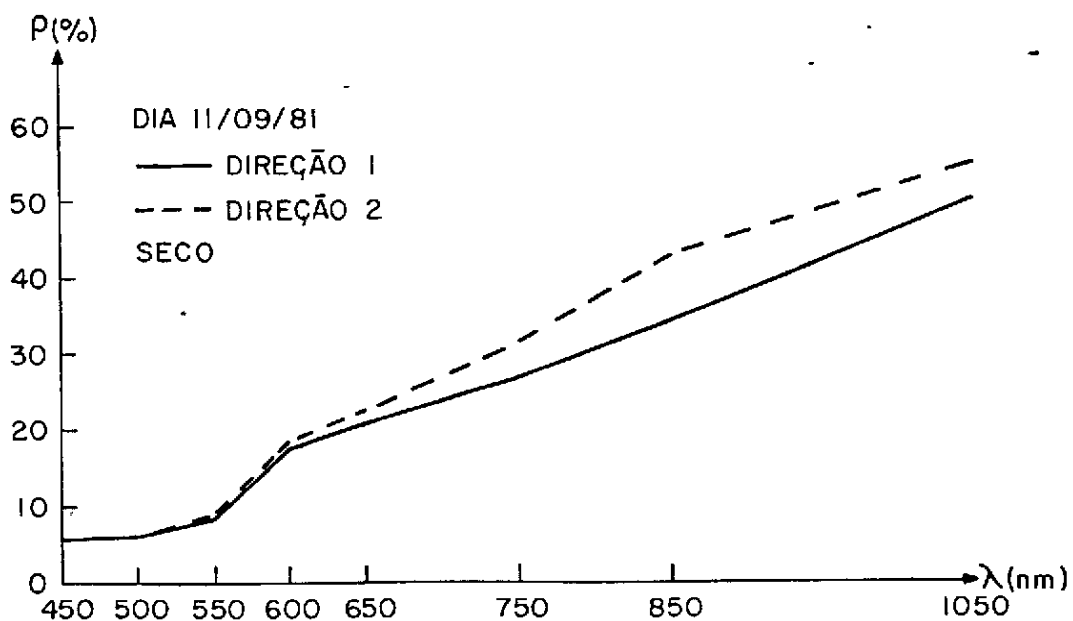
Fig. 3.1 - Comportamento espectral da parcela seca segundo as direções de observação 1 e 2 (11/09/81).
