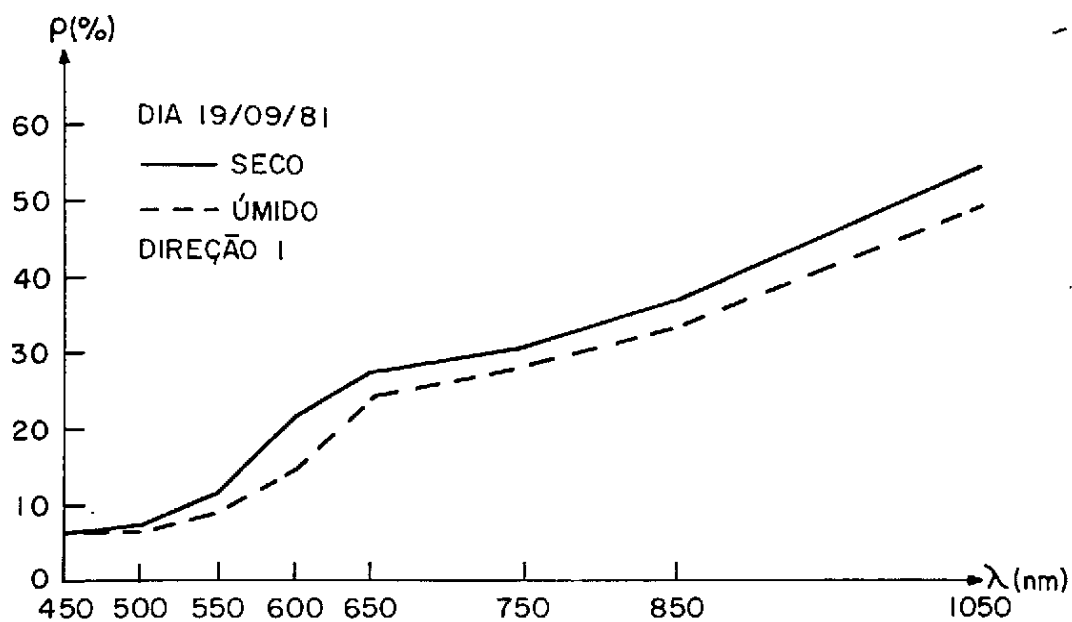
Fig. 3.24 - Comportamento espectral das parcelas seca e úmida segundo a direção de observação 1 (19/9/81).
