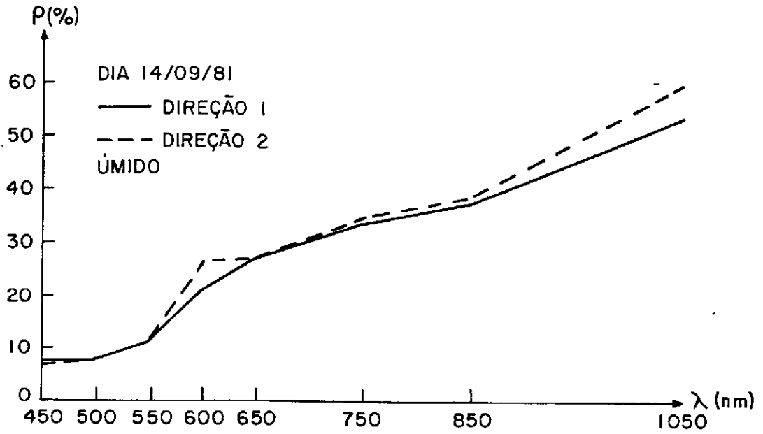
Fig. 3.9 - Comportamento espectral da parcela úmida segundo as direções de observação 1 e 2 (14/9/81).
