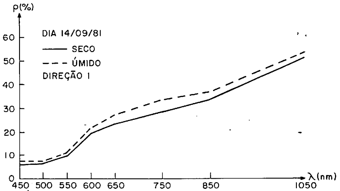
Fig. 3.15 - Comportamento espectral das parcelas seca e úmida segundo a direção de observação I (14/9/81).
