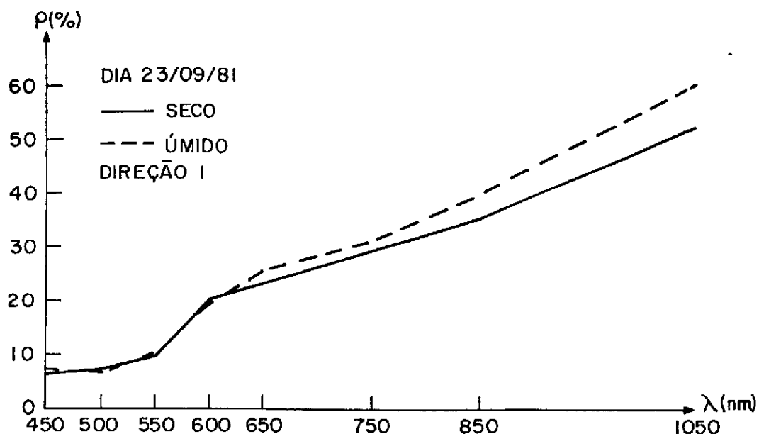
Fig. 3.28 - Comportamento espectral das parcelas seca e úmida segundo a direção de observação 1 (23/09/81).
