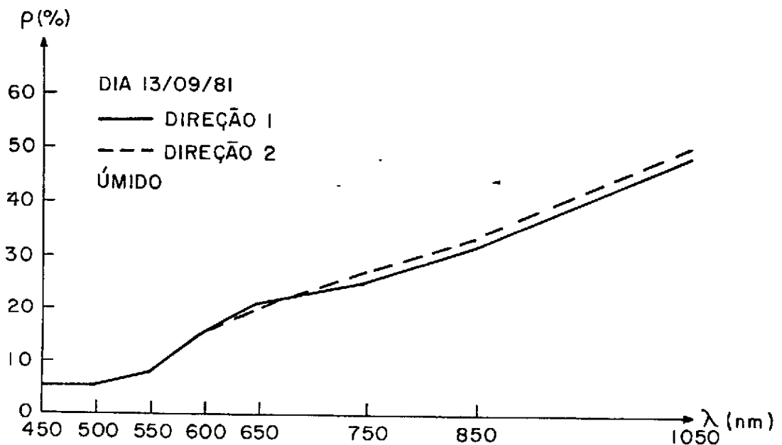
Fig. 3.8 - Comportamento espectral da parcela úmida segundo as direções de observação 1 e 2 (13/9/81).
