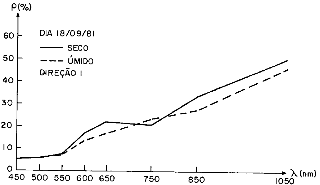
Fig. 3.23 - Comportamento espectral das parcelas seca e úmida segundo a direção de observação 1 (18/9/81).
