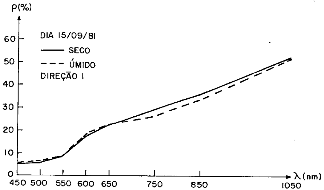
Fig. 3.16 - Comportamento espectral das parcelas seca e úmida segundo a direção de observação 1 (15/9/81).
