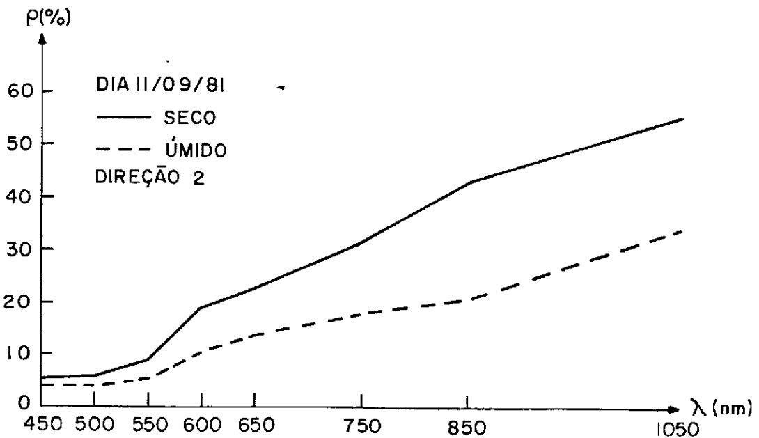
Fig. 3.17 - Comportamento espectral das parcelas seca e úmida segundo a direção de observação 2 (11/9/81) - Irrigação em 10/9/81.
