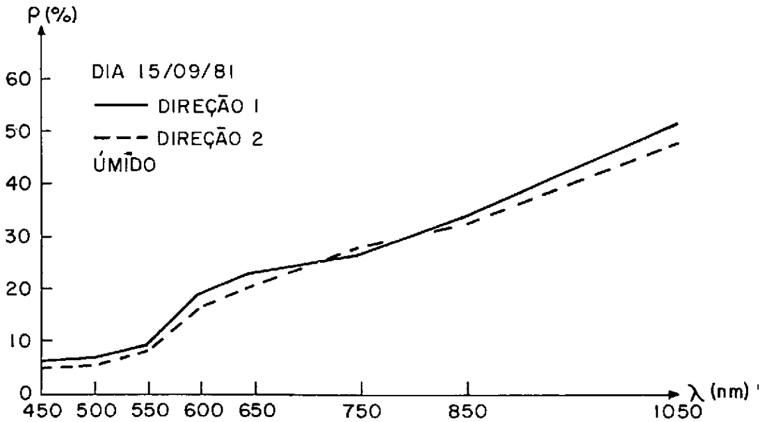
Fig. 3.10 - Comportamento espectral da parcela úmida segundo as direções de observação 1 e 2 (15/9/81).
