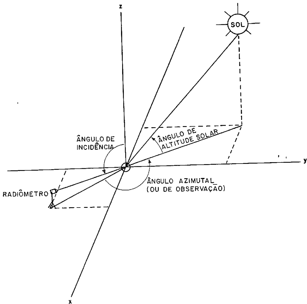
Fig. 2.2 - Ângulos envolvidos na radiometria de campo, adaptado de Egbert e Ulaby (1972).
