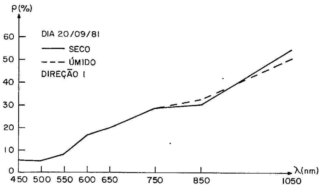
Fig. 3.25 - Comportamento espectral das parcelas seca e úmida segundo a direção de observação 1 (20/9/81).
