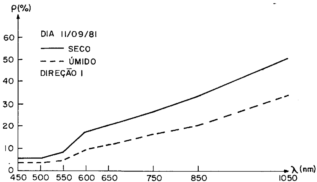
Fig. 3.12 - Comportamento espectral das parcelas seca e úmida segundo a direção de observação I (11/9/81) - Irrigação em 10/9/81.
