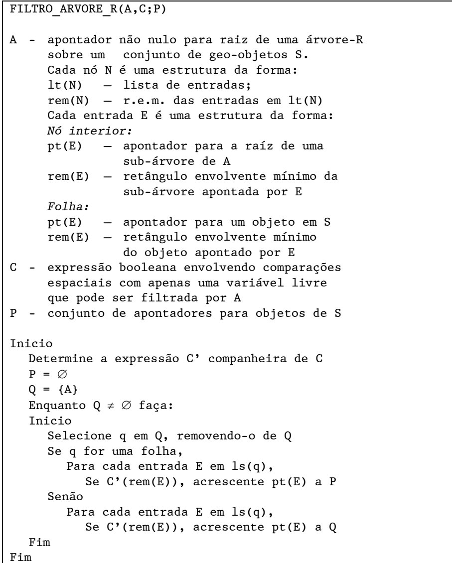
Figura 7.5 – Filtro por árvores-R.
