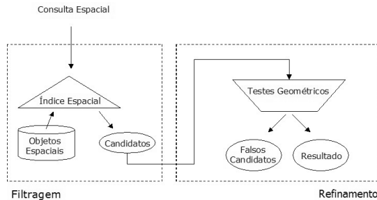
Figura 6.3 – Processamento de consultas espaciais. Fonte: adaptada de Gaede e Günther (1998).
