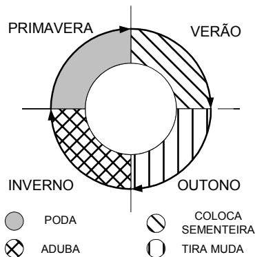
Figura 4.3 – Tempo circular.
