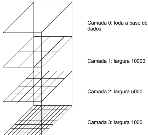
Figura 6.15 – Tiling.
