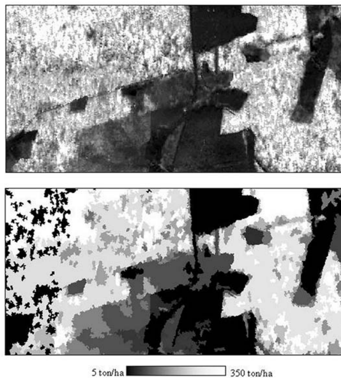
Figura 4. Seção de imagem interferométrica SAR (bandas X e P) e mapa da distribuição de cobertura florestal correspondente em área do Tapajós
