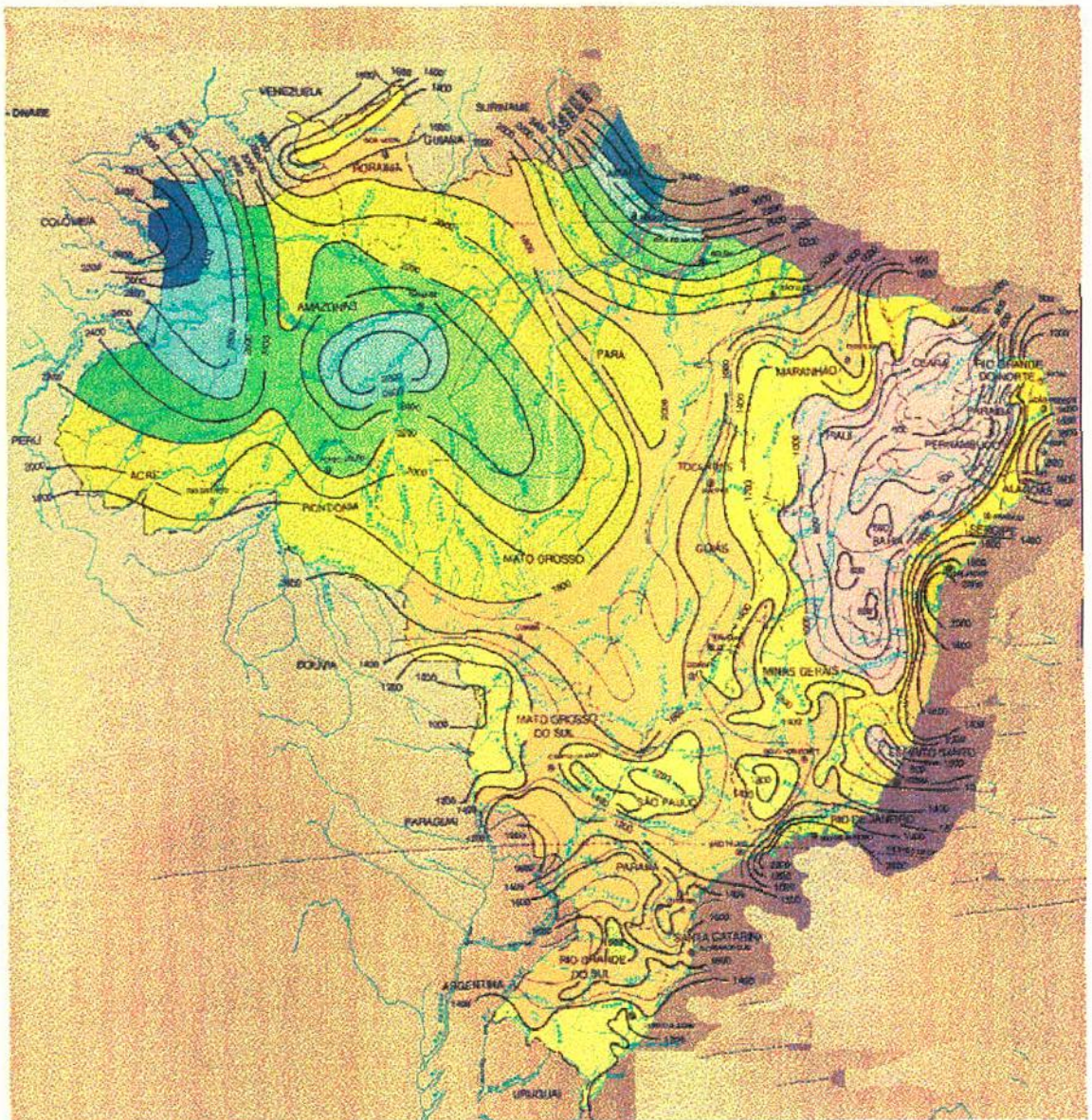
Fig. 5 - Mapa indicativo que representa a superposição do Mapa MIR sobre o Mapa das Isoietas Médias Anuais do Brasil
