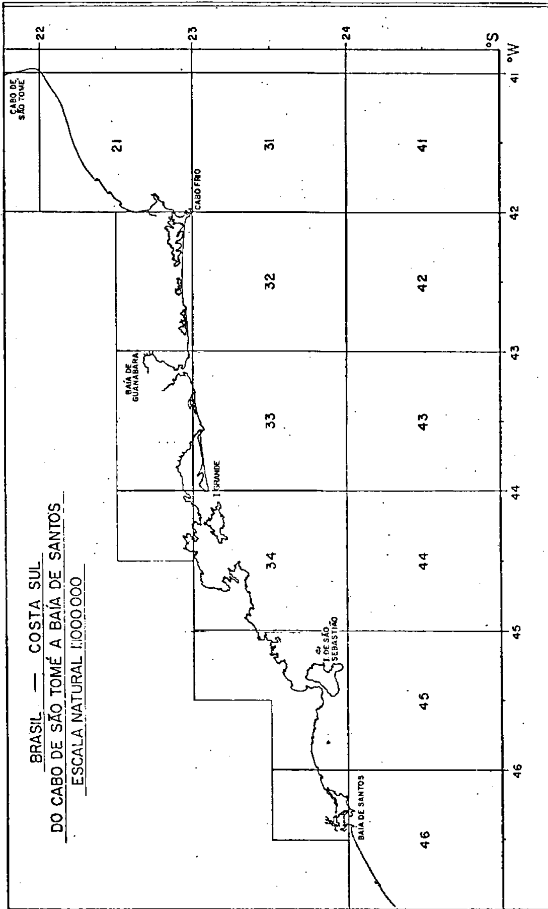
Fig. II.3 - Área teste e os quadrados de 1° x 1° do Quadrado de Marsden nº 376 na costa
