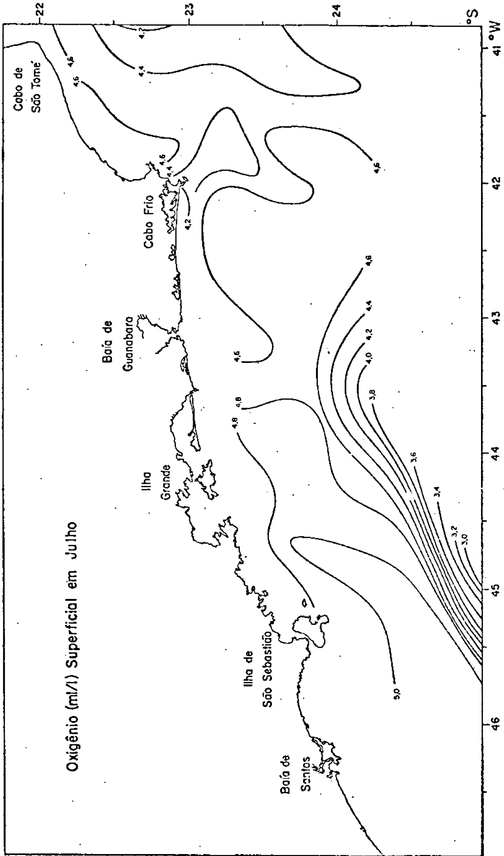
Fig. III.3 - Distribuição do oxigênio (ml/l) superficial em Julho
