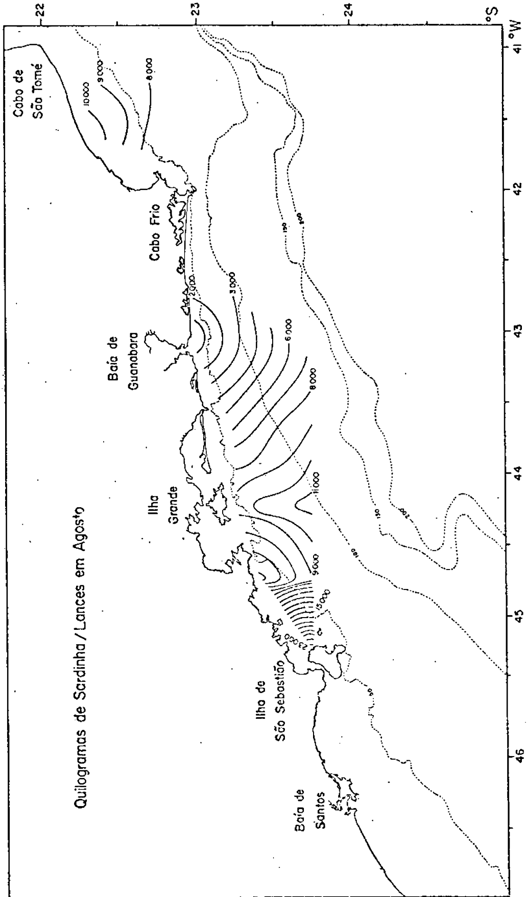
Fig. III.10 - Distribuição da captura de sardinha (kg/lance) em Agosto
