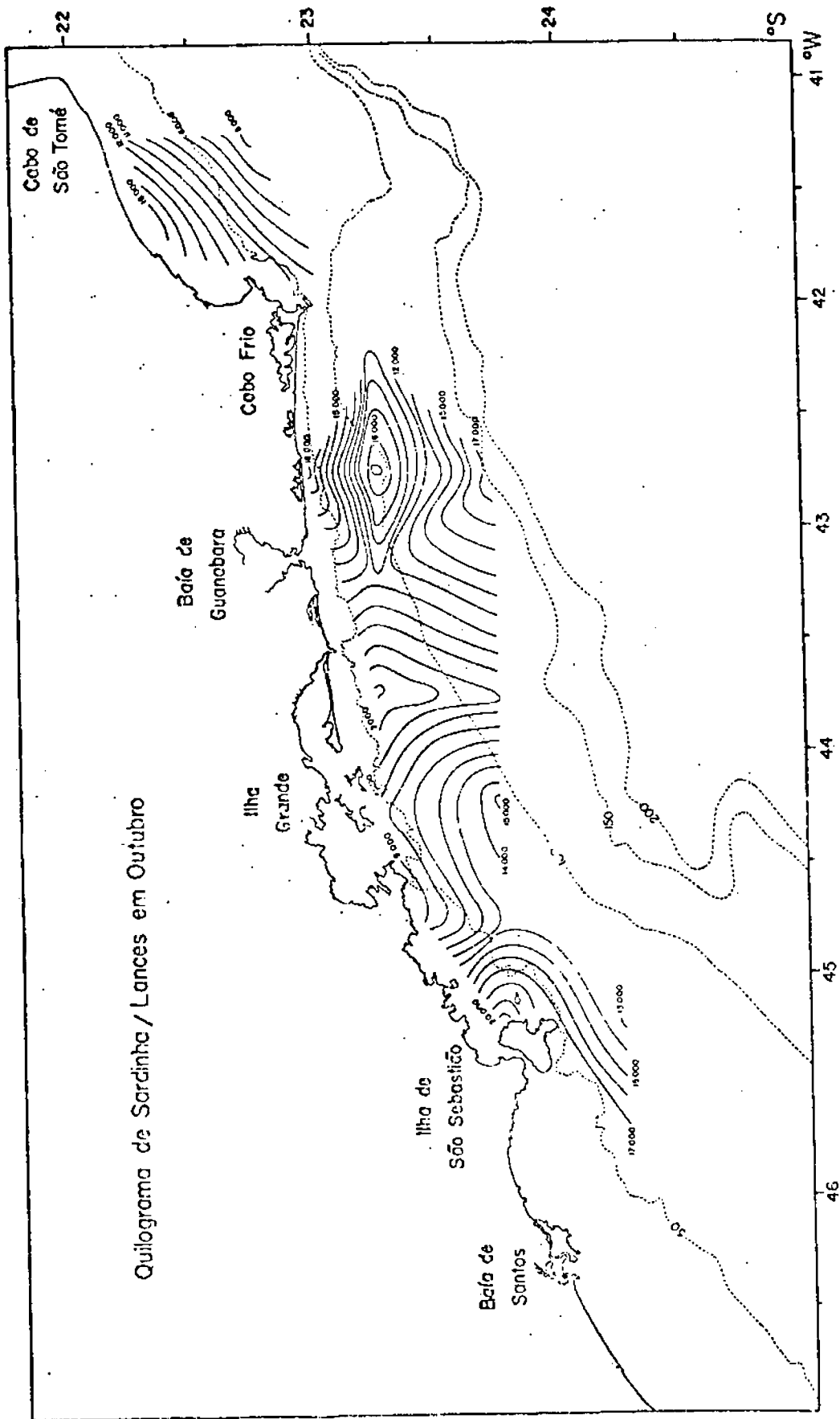
Fig. III.21 - Distribuição da captura de sardinha (kg/lance) em Outubro
