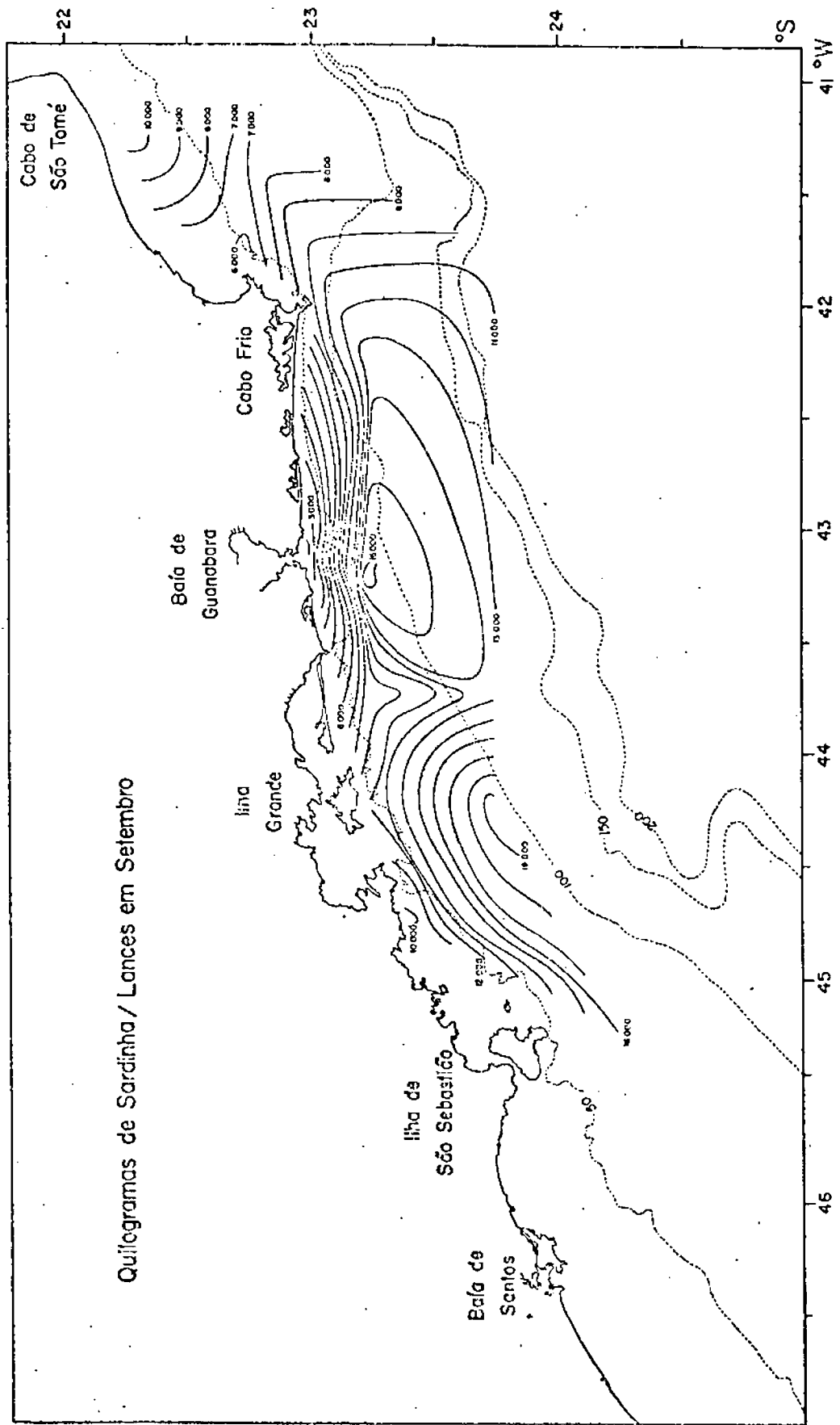
Fig. III.16 - Distribuição da captura de sardinha (kg/lance) em Setembro
