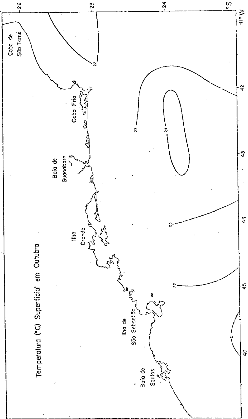
Fig. III.17 - Distribuição da temperatura (°C) superficial em Outubro
