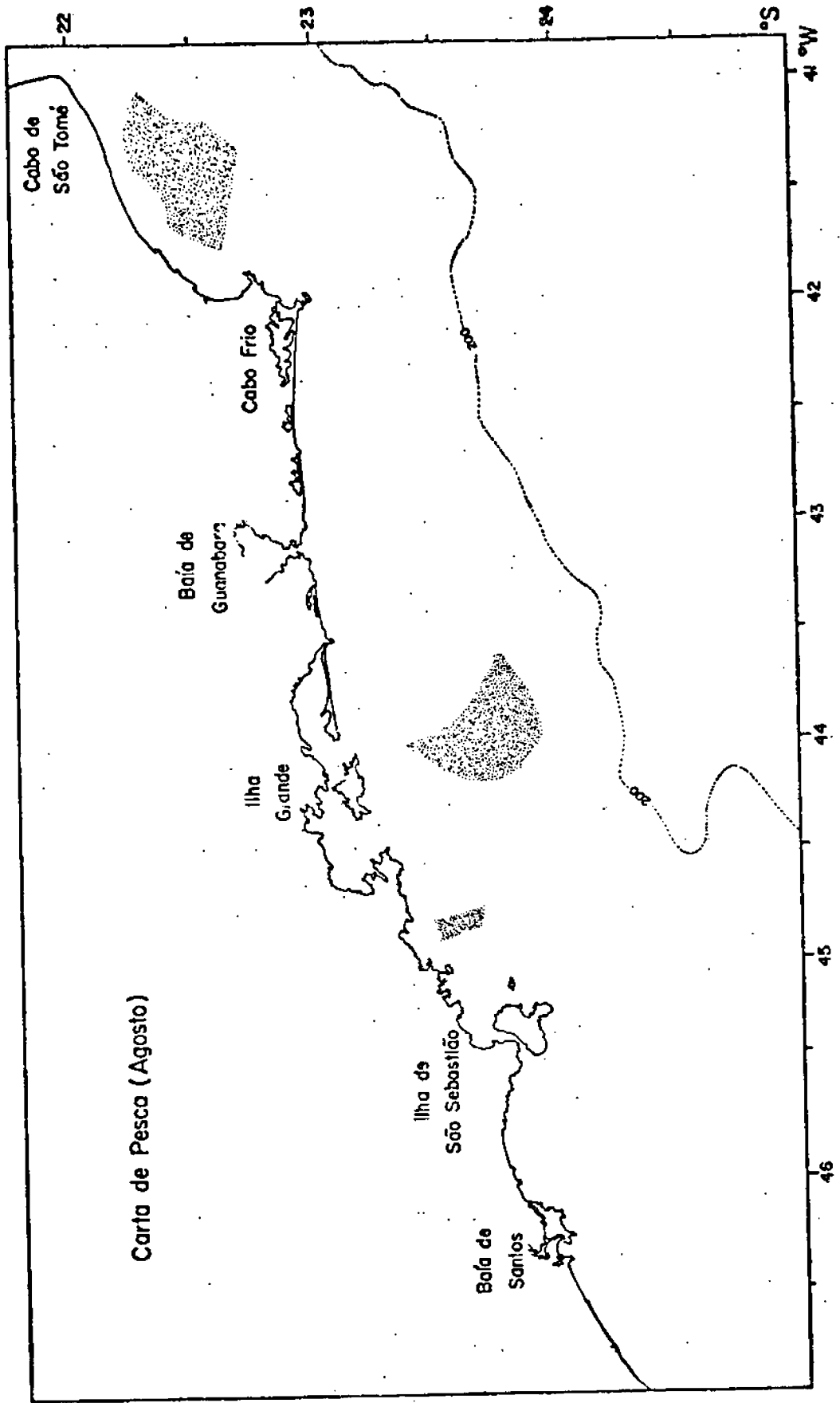
Fig. IV.12 - Carta de Pesca em Agosto
