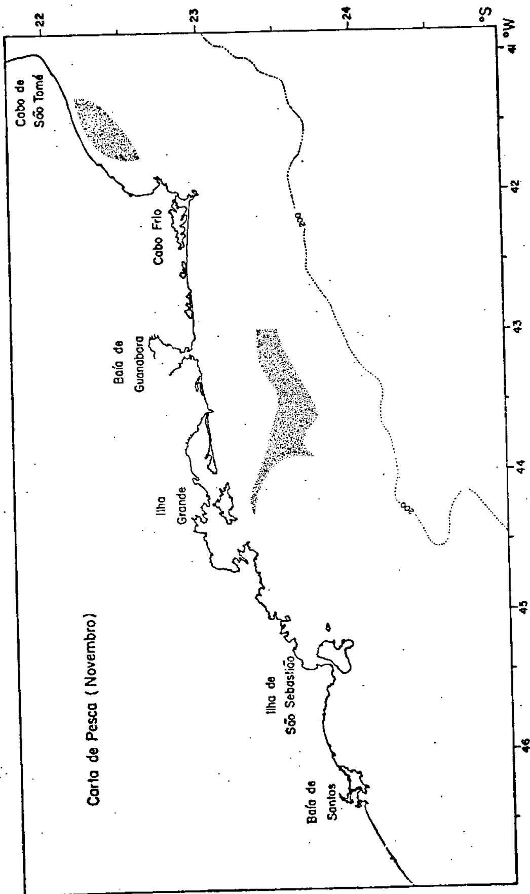
Fig. IV.14 - Carta de Pesca em Novembro
