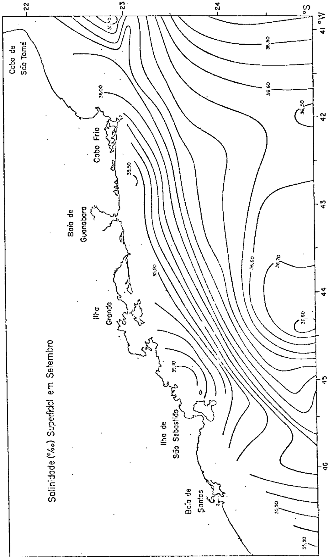
Fig. III.12 - Distribuição da salinidade (‰) superficial em Setembro
