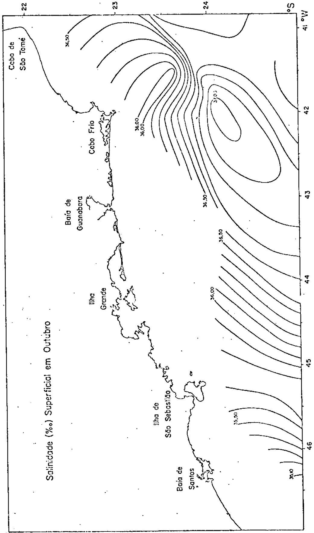
Fig. III.18 - Distribuição da salinidade (‰) superficial em Outubro
