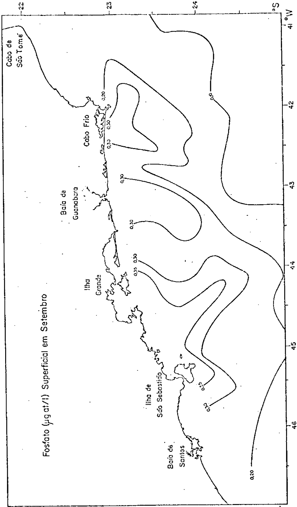
Fig. III.14 - Distribuição do fosfato ( \mu\text{g at/l} ) superficial em Setembro
