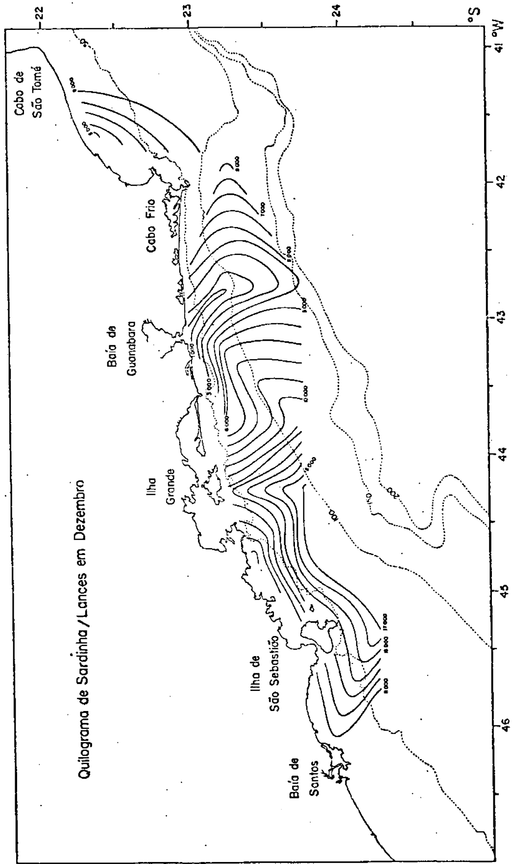
Fig. III.31 - Distribuição da captura de sardinha (kg/lance) em Dezembro
