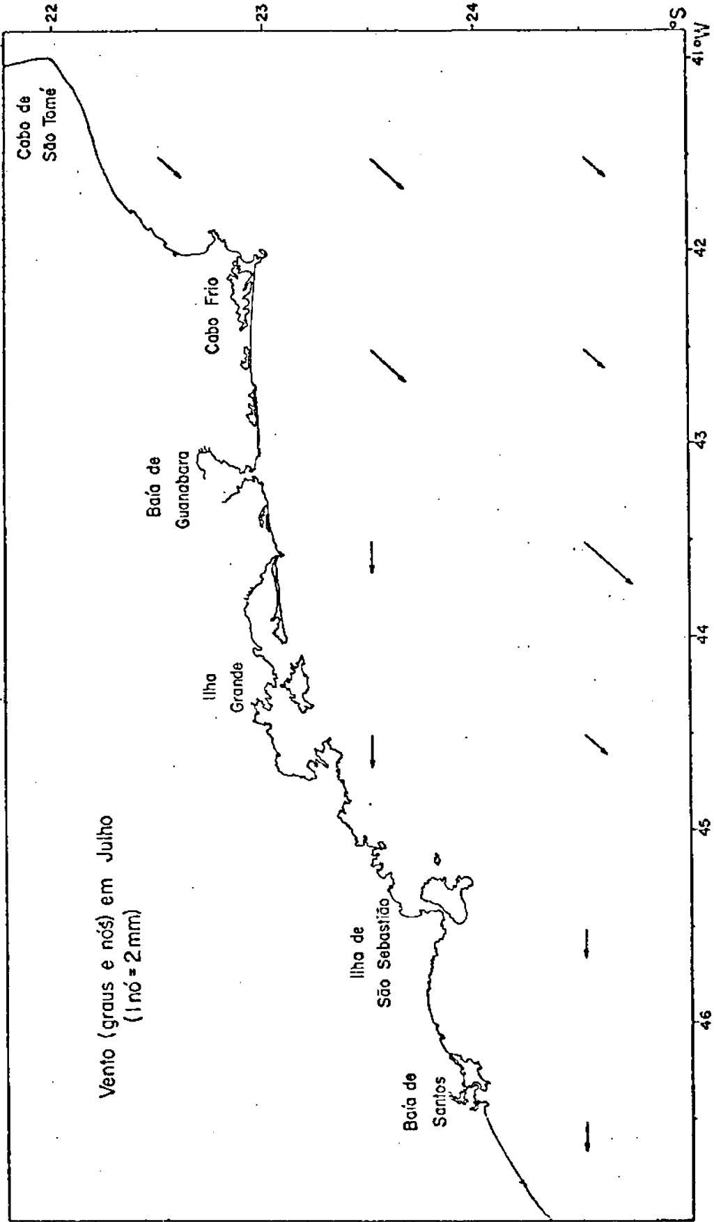
Fig. III.4 - Distribuição do vento (graus e nós) em Julho
