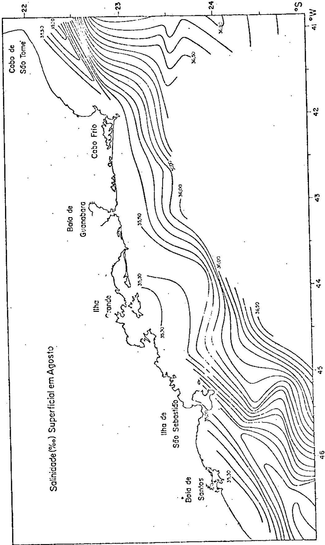
Fig. III.7 - Distribuição da salinidade (‰) superficial em Agosto
