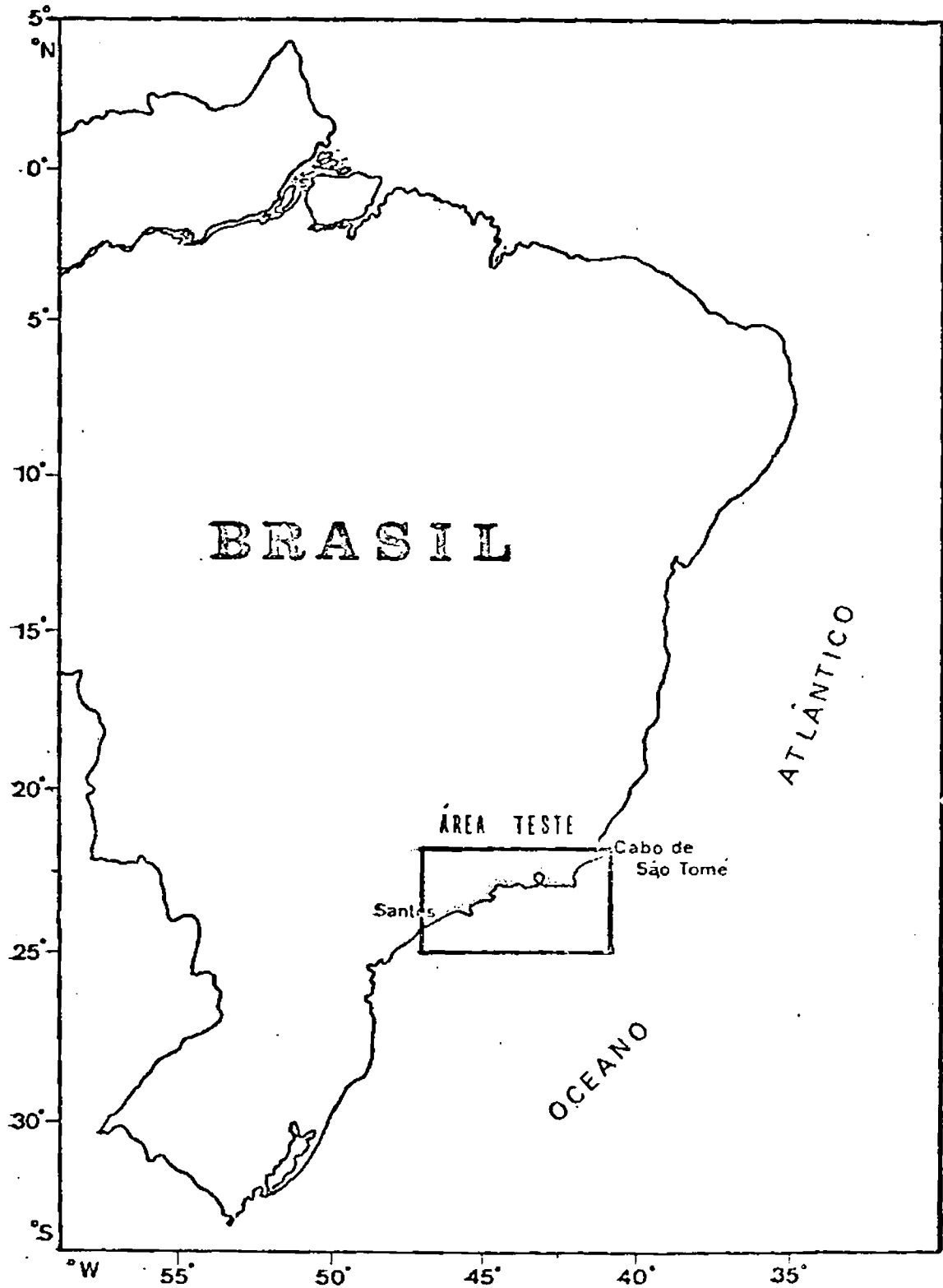
Fig. I.1 - Localização da área teste
