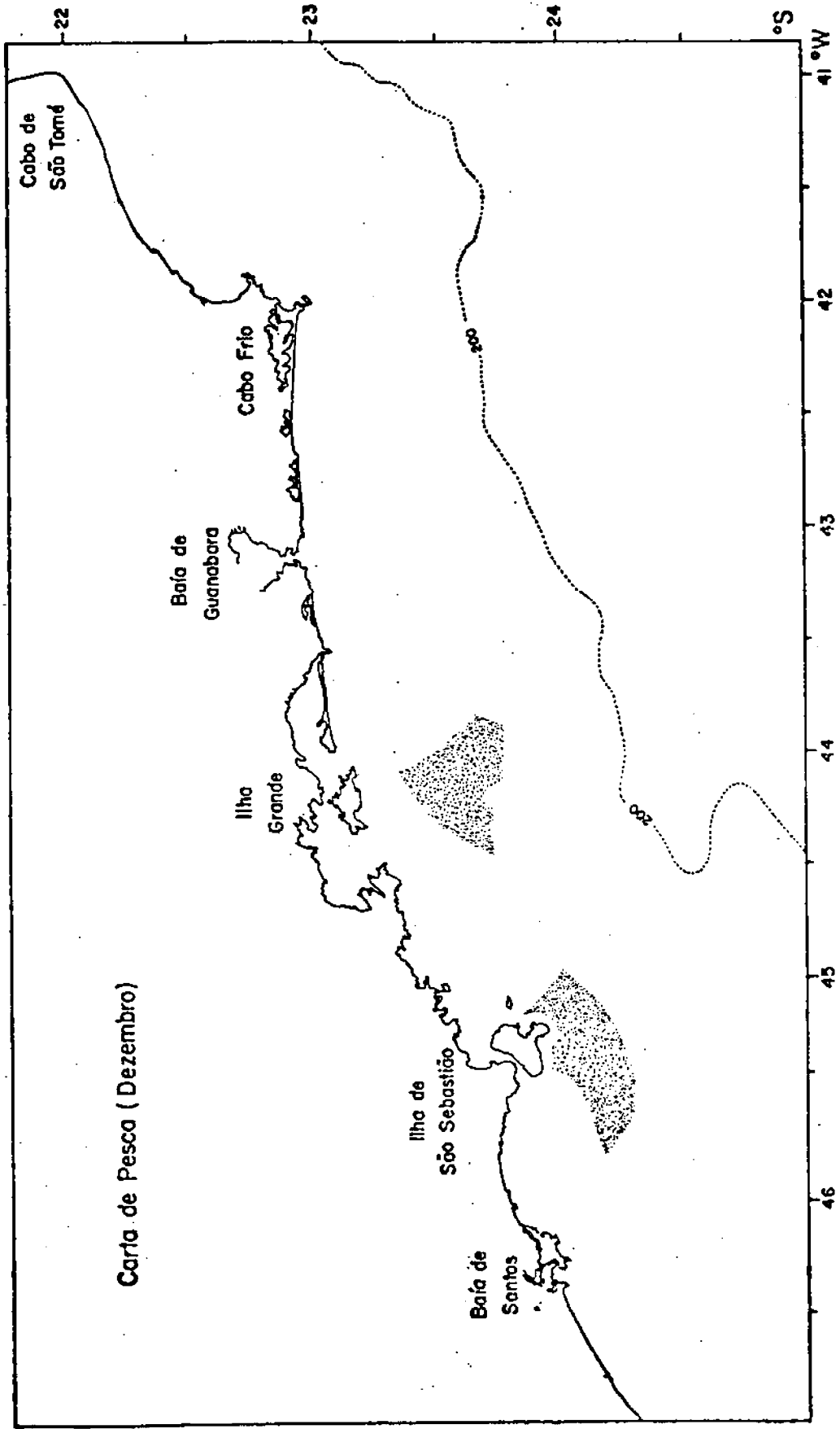
Fig. IV.15 - Carta de Pesca em Dezembro
